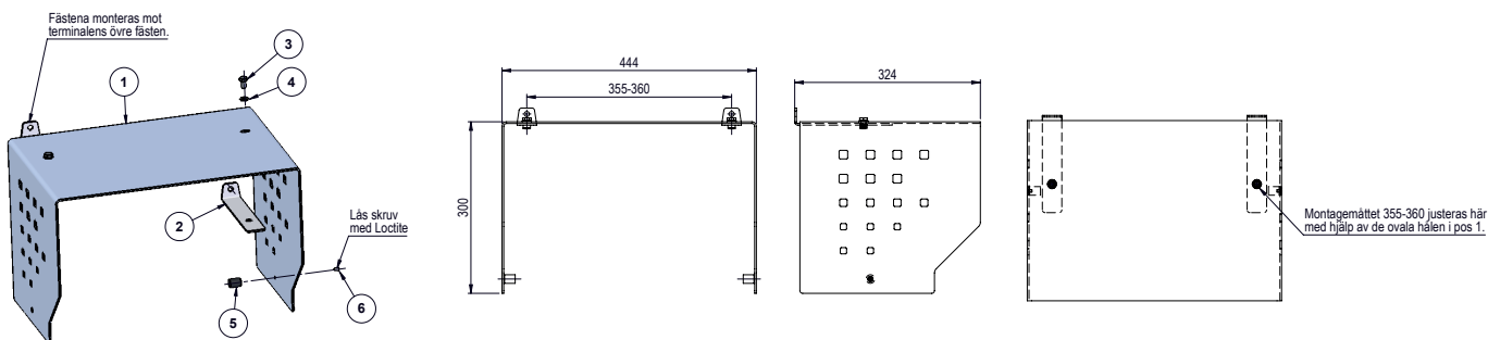
1. Vädterskydd | 2. Konsol | 3. Sexkantskruv | 4. Bricka | 5. Gummidämpare | 6. Förs. krysskruv
